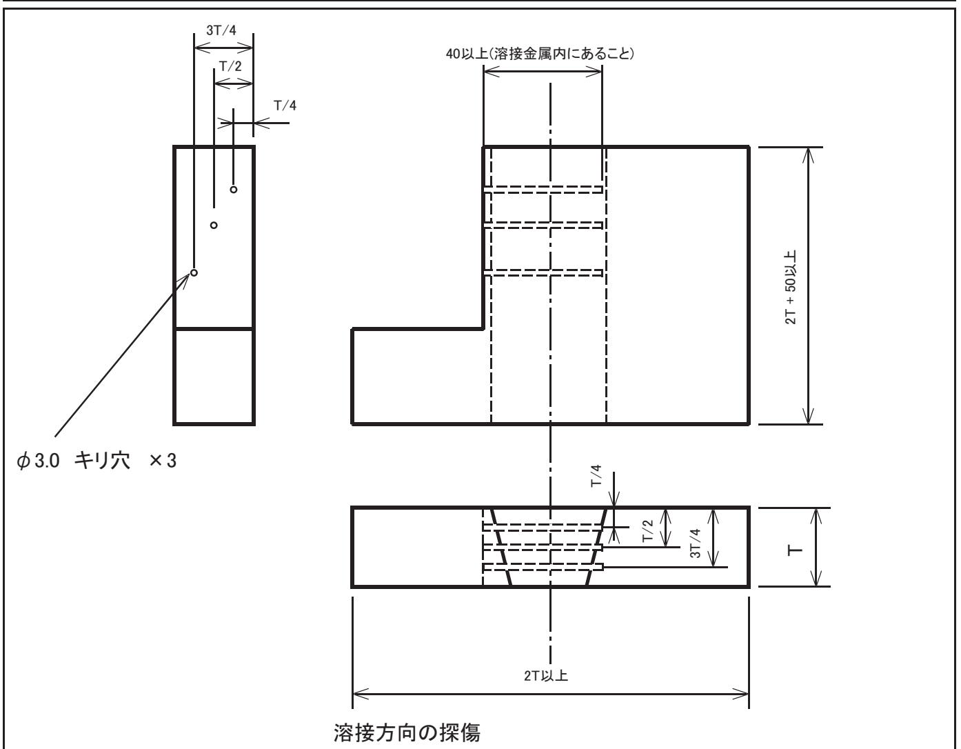
図3(a) RB-W (板厚25mmを超える場合)
