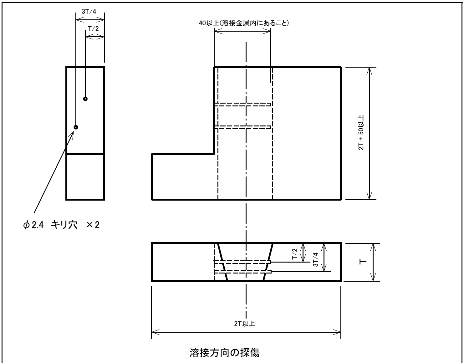
図3(b) RB-W (板厚9mm以上25mm以下の場合)
